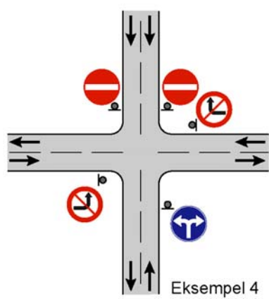
Figur 2.3 Eksempler på anvendelse av skilt 402
