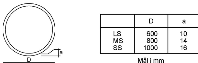
Fig. 2.2 Påbudsskilt - størrelse og utforming
