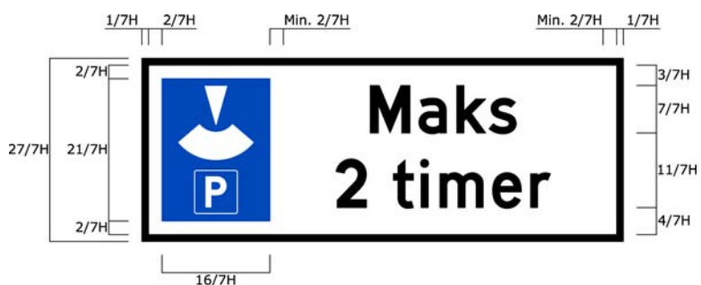
Figur 4.25b Utforming av underskilt 831
