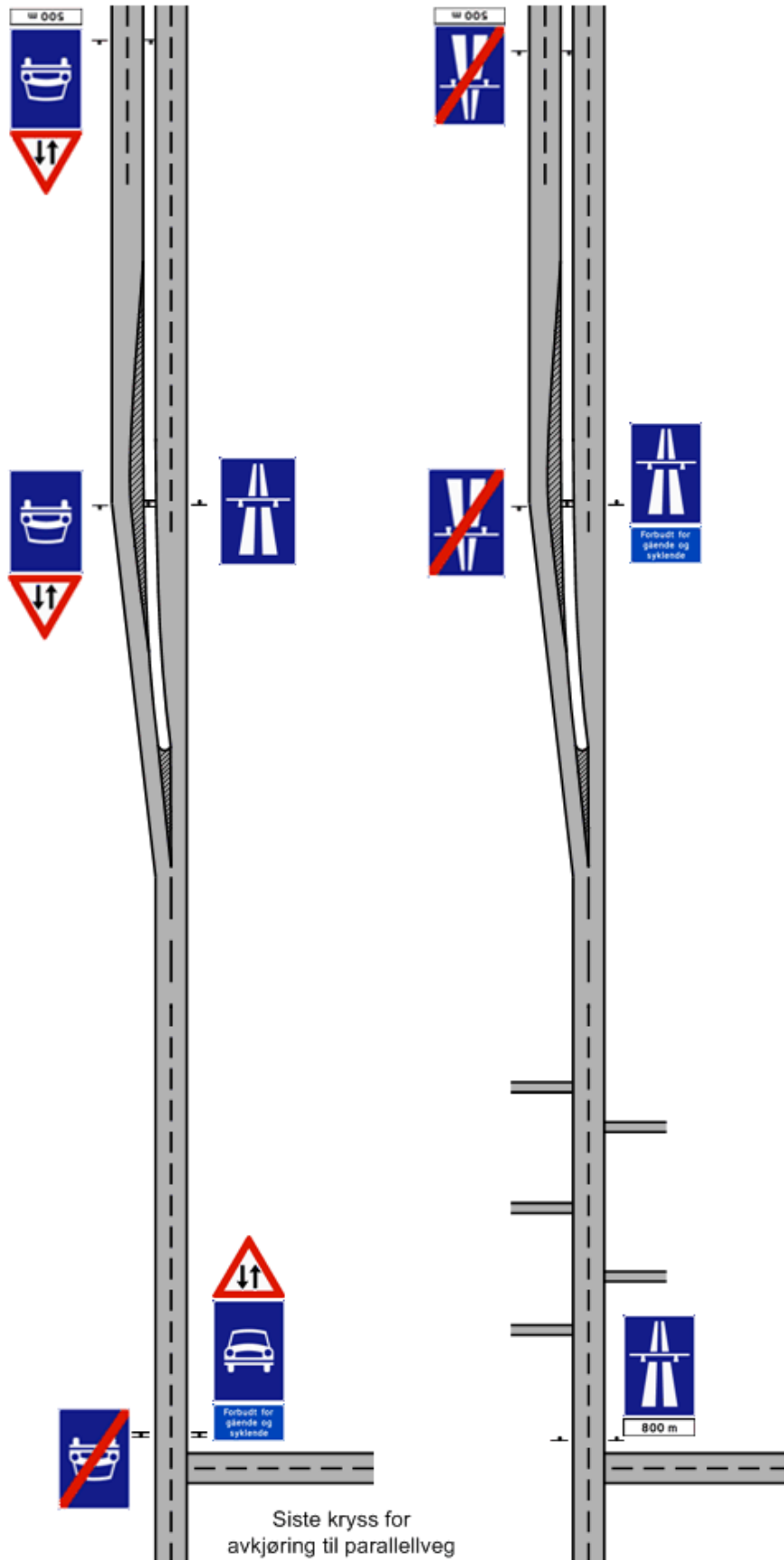
Figur 3.3 Eksempler på forvarsling og skilting av motorveg
