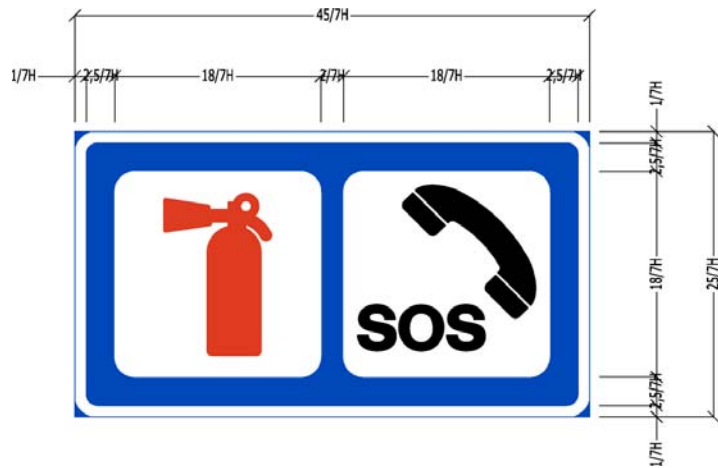
Figur 3.20 Utforming av skilt 600.21H når det står sammen med skilt 555 i størrelse US (avvik fra normalutformingen for serviceskilt)
