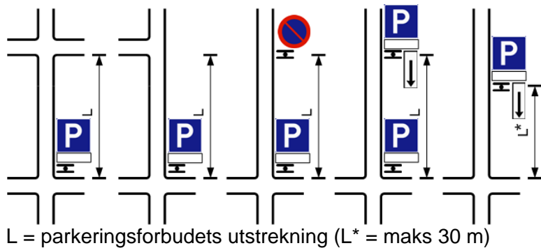
Figur 1.14 Eksempler på utstrekning av regulering med skilt 552
