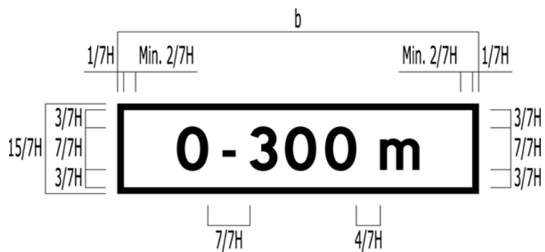
Figur 4.6 Plassering av tekst på underskilt 804
