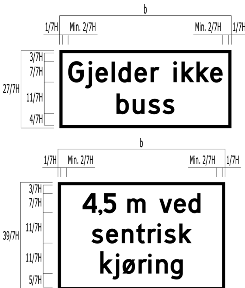
Figur 4.19 Plassering av tekst på underskiltene 808.311-333, 808.341 og 808.351
