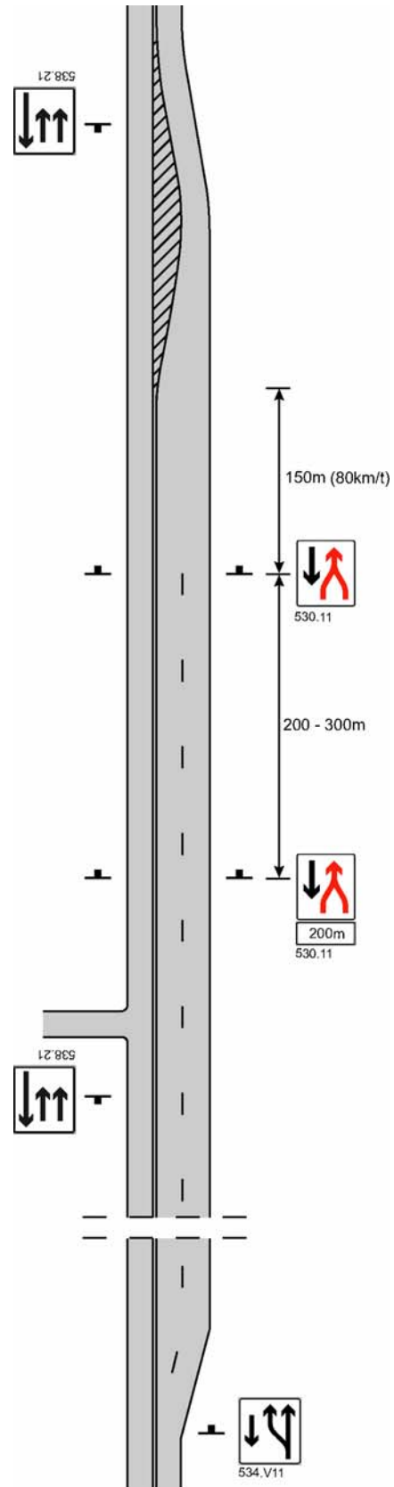
Fig. 3.12 Skilting av forbikjøringsfelt
