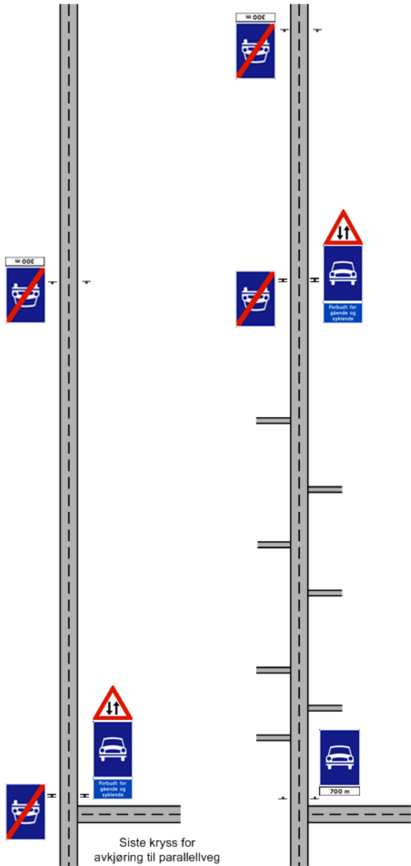
Figur 3.4 Eksempler på forvarsling og skilting av motortrafikkveg
