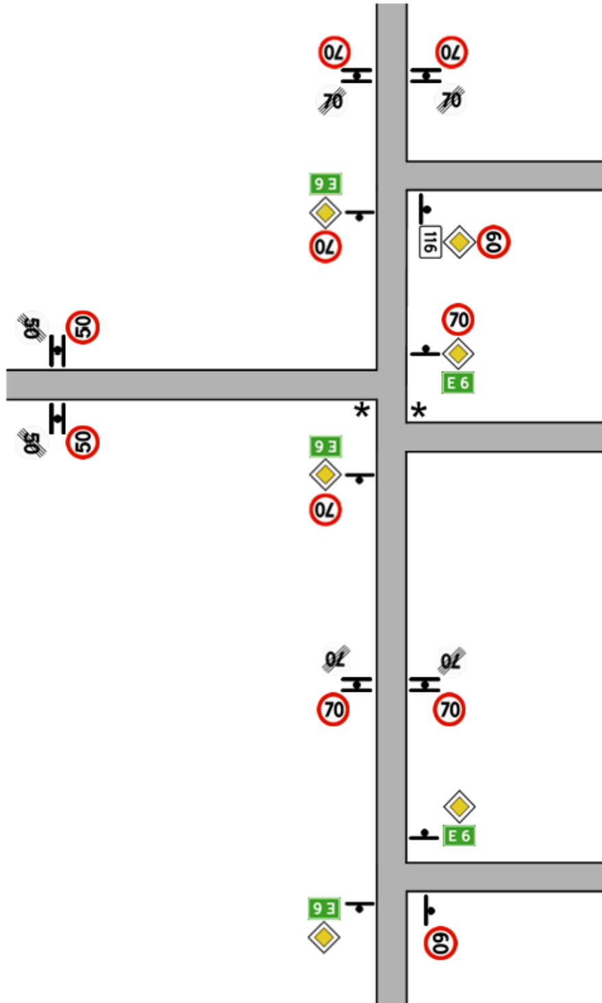
Figur 1.6 Eksempel på skilting av fartsgrenser utenfor tettbygd strøk
