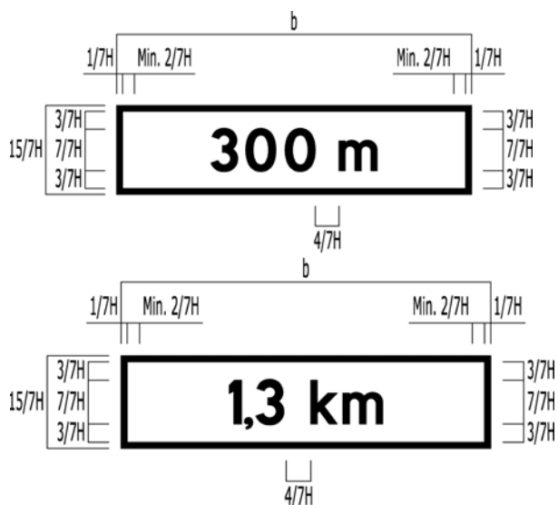
Figur 4.4 Plassering av tekst på underskilt 802
