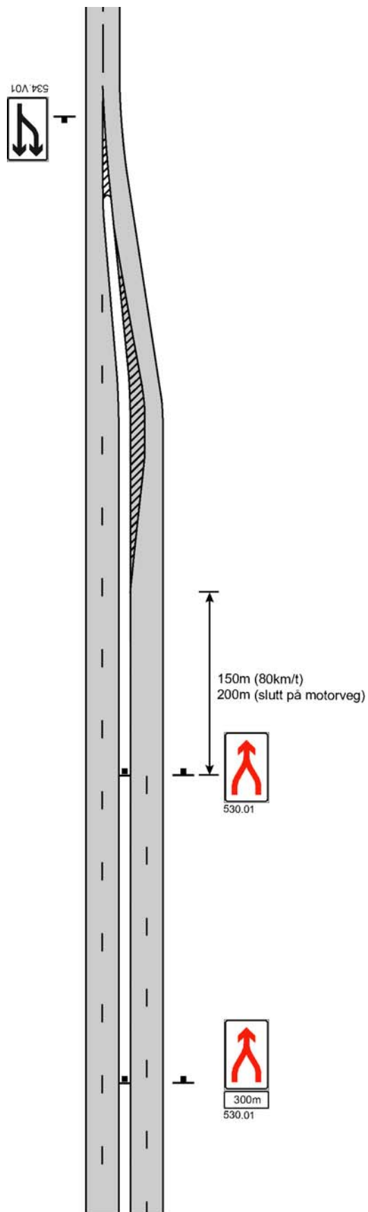
Fig. 3.14 Skilting av overgang mellom firefelts og tofelts veg ( V \geq 80 km/t)
