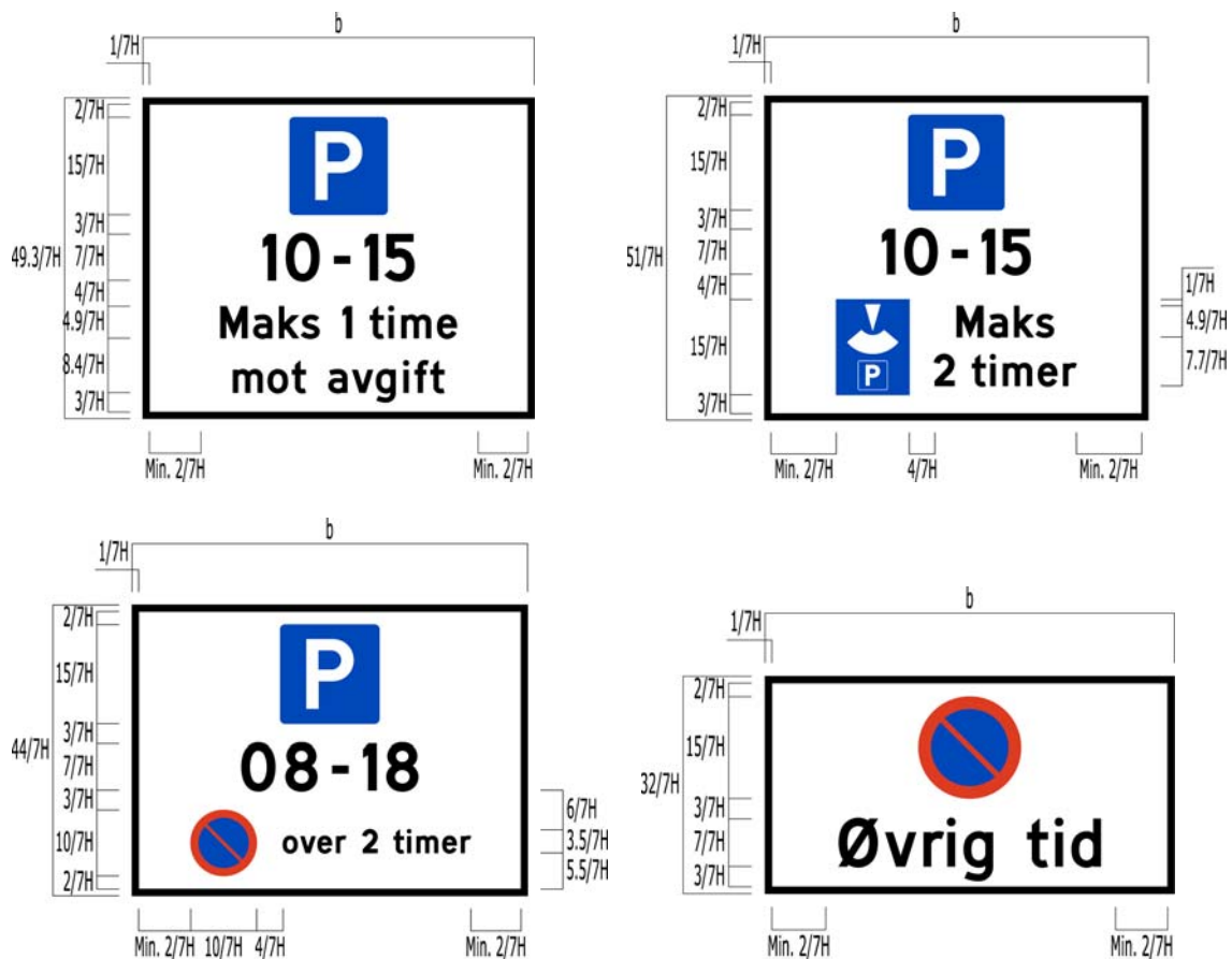
Figur 4.29 Utforming av underskilt 834 når det brukes til skilt 370 og 372
