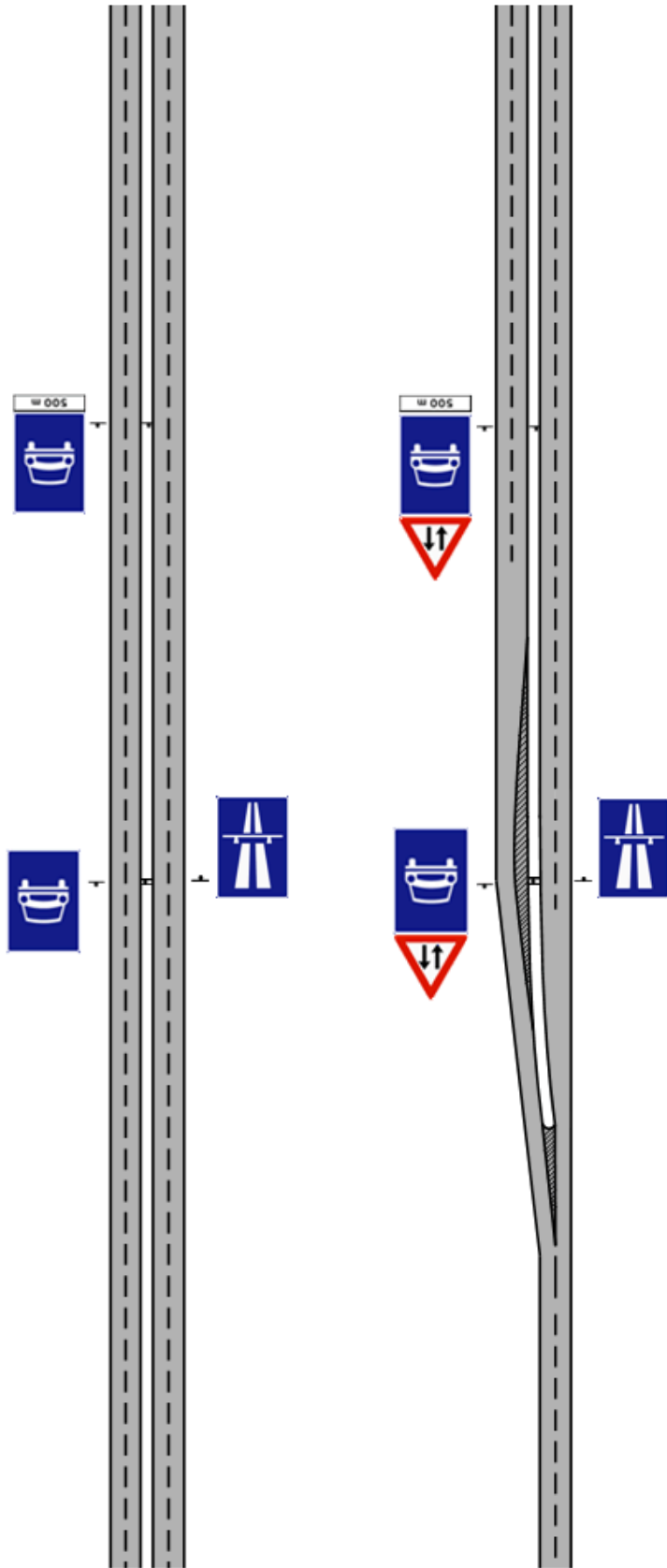
Figur 3.5 Skilting av overgang mellom motorveg og motortrafikkveg
