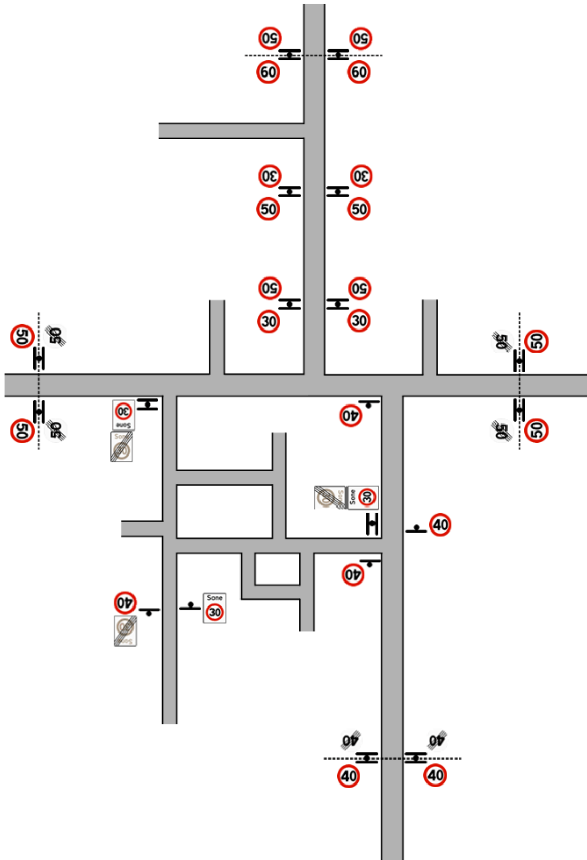
Figur 1.7 Eksempler på skilting av fartsgrenser i tettbygd strøk
