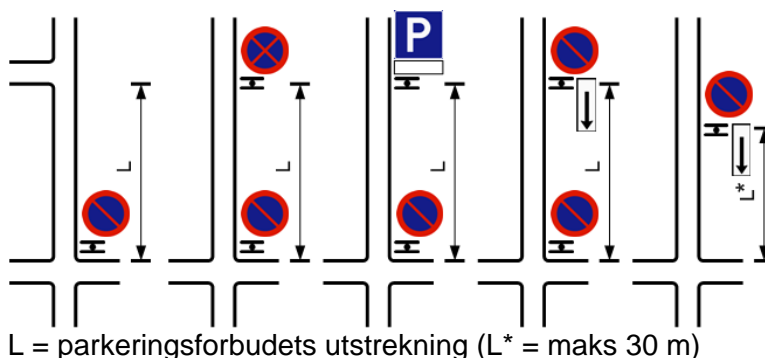
Figur 1.11 Eksempler på utstrekning av parkeringsforbud med skilt 372
