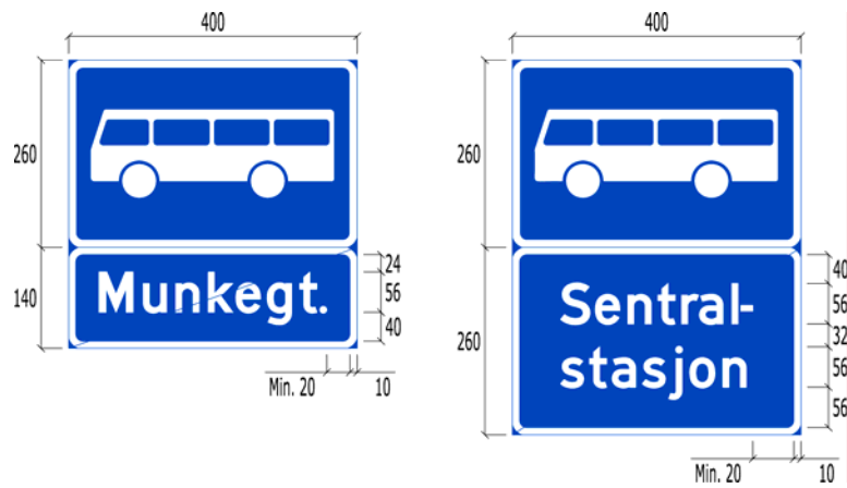
Figur 3.7 Utforming av stedsnavnskilt med holdeplassnavn
