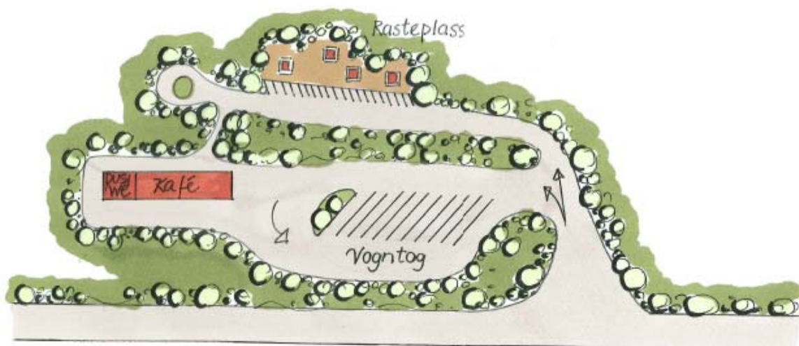
Figur 12 Eksempel på minimumsløsning (for mer trafikksvake områder). 10 oppstillingsplasser i tilknytning til rasteplass/vegkro. Tungbilplassene fysisk atskilt fra personbiler.
