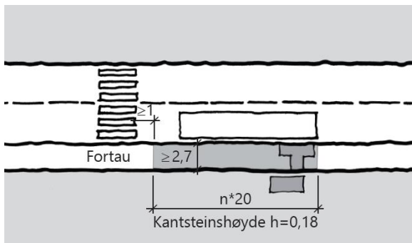
Figur D.36: Kantslipp for buss, n angir antall busser som forventes å stoppe samtidig (mål i m)
