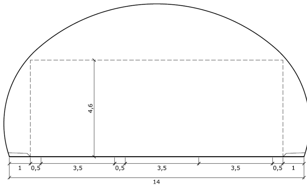
Figur V1.7 Tunnelprofil T14 med forsterket midtoppmerking og forbigjøringsfelt (mål i m).
