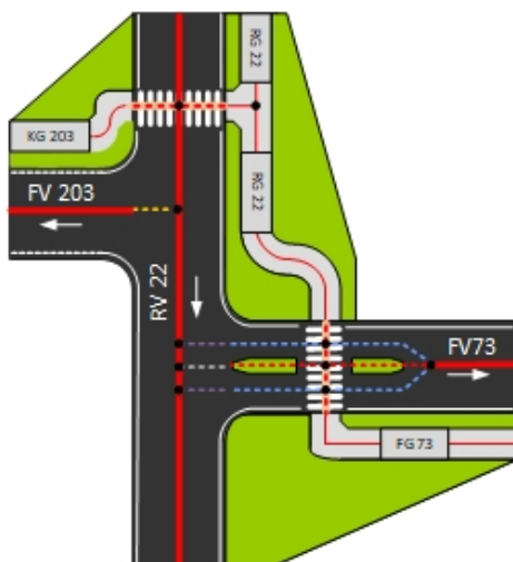
Figur 77: Gang- og sykkelvegens vegkategori gjenspeiler hvem som har forvaltningsansvaret for vegen, vegstatus G viser at dette er gs-veg og vegnummer gjenspeiler vegnummeret på den vegen gs-vegen fører trafikk for.
