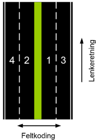
Figur 51: Feltkoden gir oss informasjon om kjørefeltene i vegens tverrsnitt.
