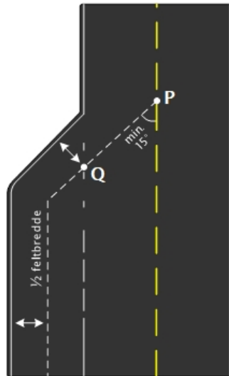
Figur 50: Konnekteringslenke for rampe..
