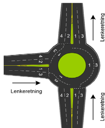
Figur 59: Rundkjøring med flere felt.
