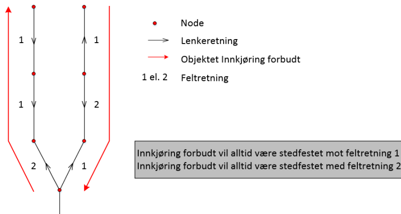
Figur 56: Eksempel som viser forholdet mellom lenkeretning, feltnummerering og innkjøring forbudt
