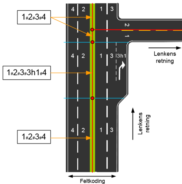
Figur 52: Feltoversikt. Rammene til venstre i figuren viser feltstrekningsobjektets koding av felt.
