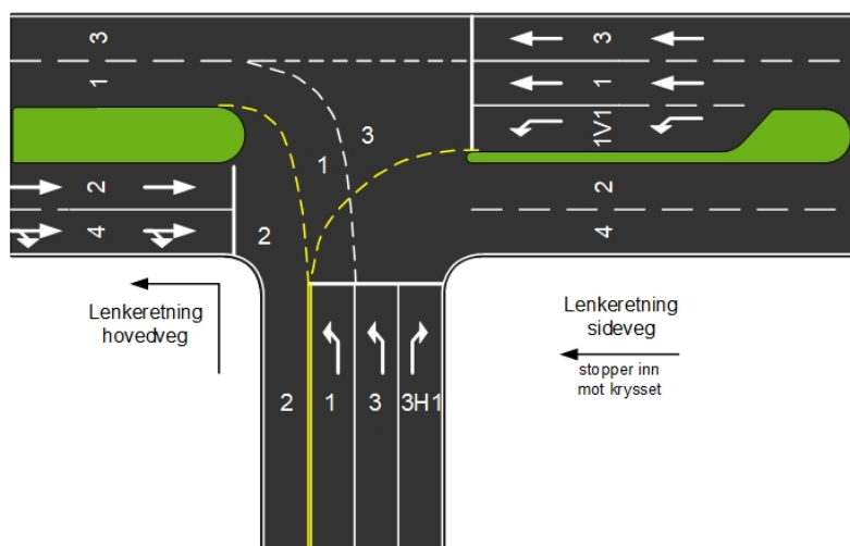
Figur 69: Eksempel på et kryss hvor hovedvegen gjør en 90° sving, også kalt stjernekruss.
