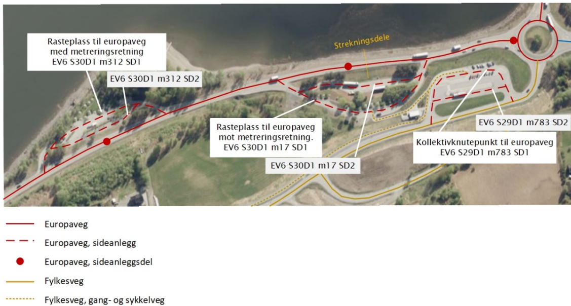
Figur 45: Metring av sideanlegg
