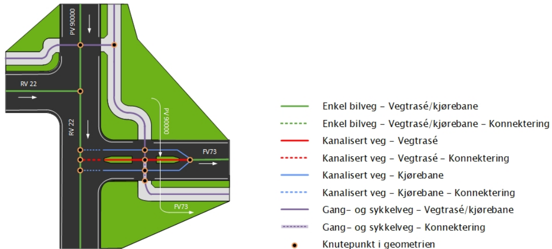
Figur 32: Geometrien skal splittes i alle geometriknutepunkt mellom gs-veg og kjøreveg.
