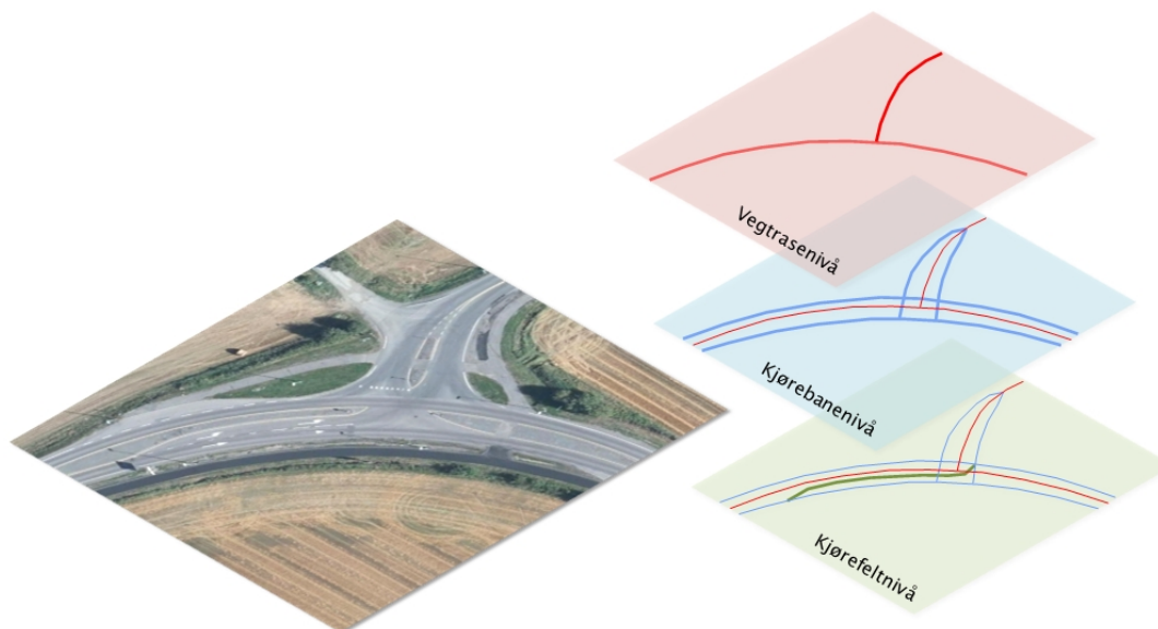
Figur 18: Et vegkryss betraktet på vegtrasénivå (øverst), kjørebanelnivå og kjørefeltnivå.
