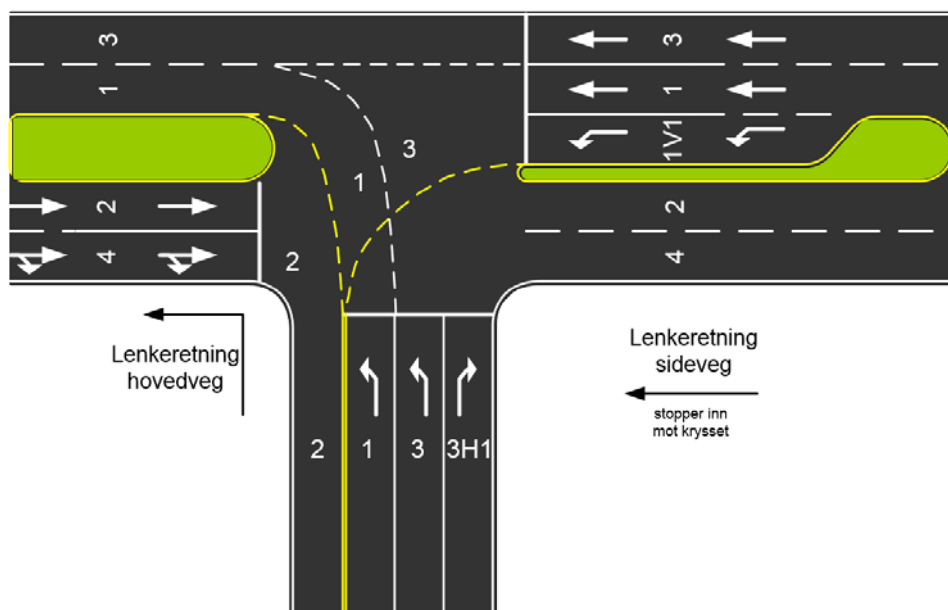
Figur 62: Svingefelt i kryss med 90°metrering.
