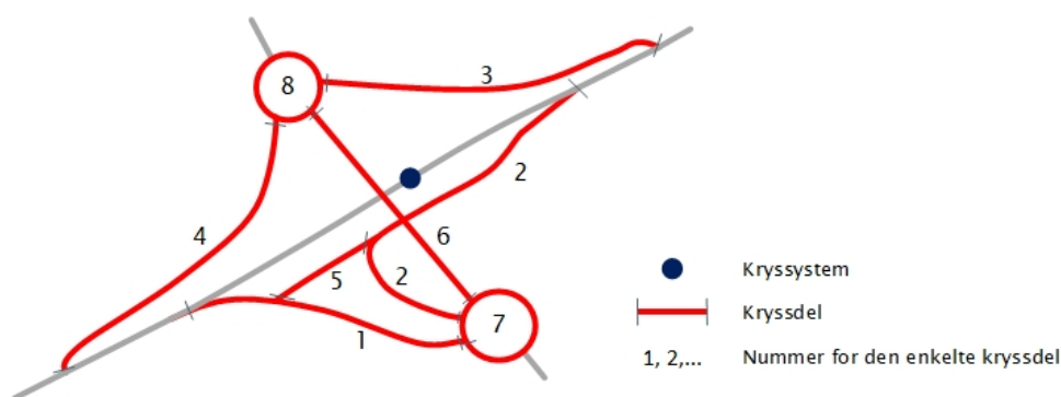
Figur 42: Grafisk fremstilling av et kryssystem.
