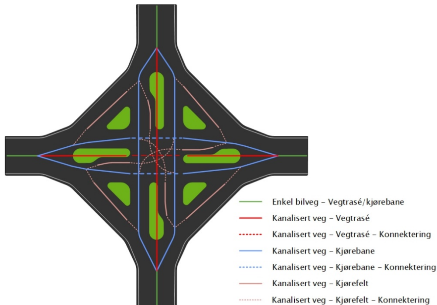
Figur 25: Geometri i kryss, alle nivåer.
