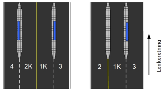
Figur 65: Kollektivfelt i felt 1. Pilen angir lenkeretningen for begge eksemplene.
