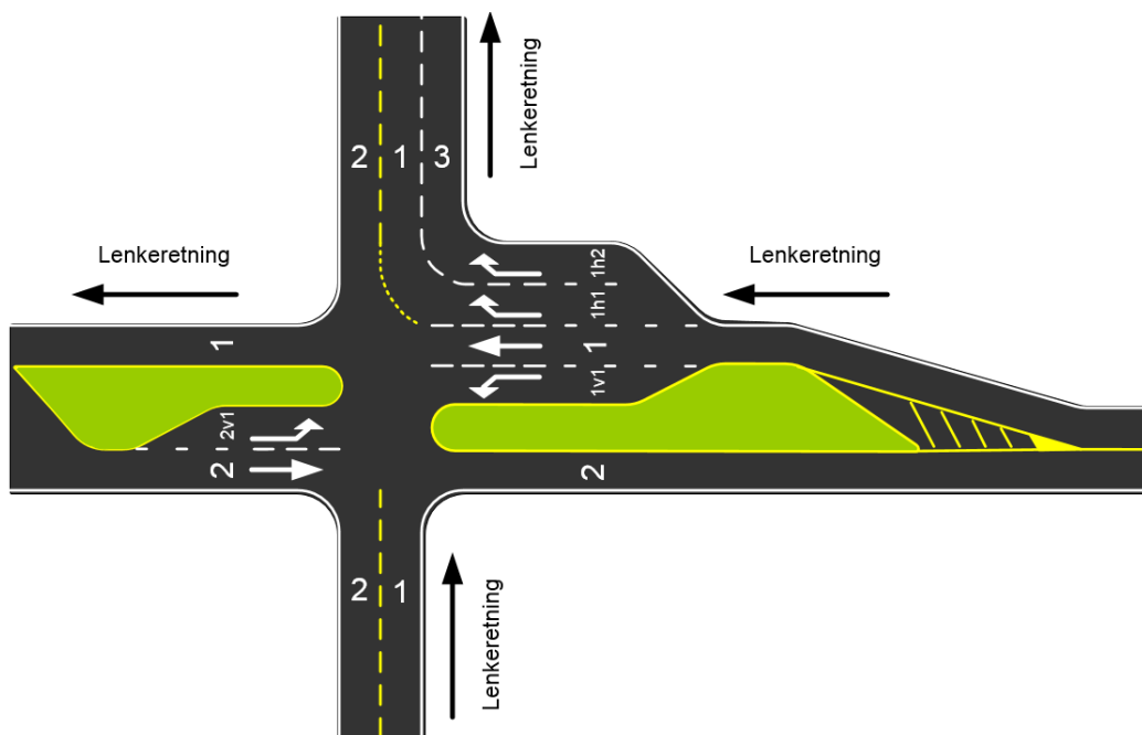
Figur 61: Svingefelt på hovedvegen går over til å bli hovedfelt på sidevegen.
