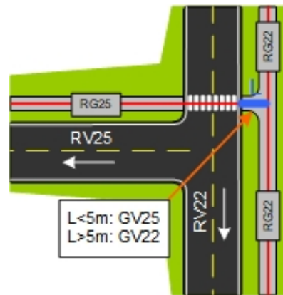
Figur 79: Om en liten strekning mellom to gang- og sykkelveger skal høre til den ene gs-vegen eller den andre avgjøres av lengden på strekningen. Dersom denne strekningen (markert som L i figuren) er kortere enn 5 meter, skal den metrerer sammen med den tilstøtende gs-veg.
