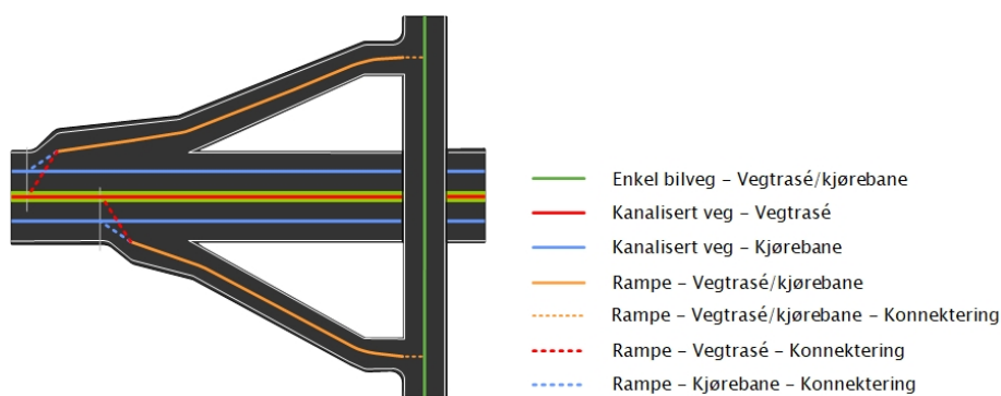
Figur 27: Geometri i planskilt kryss med rampesystem.
