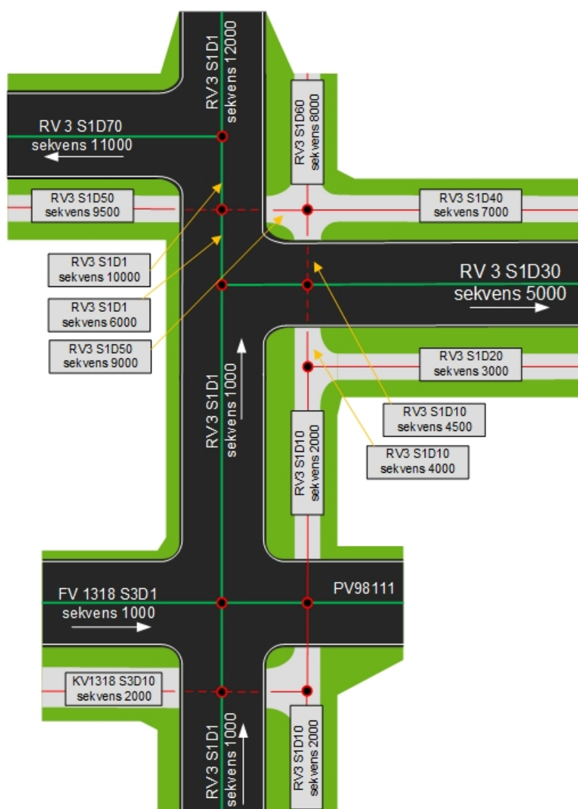
Figur 68: Eksempel på sekvensnummerering
