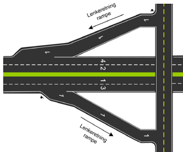
Figur 60: Ramper består ofte av et felt for trafikk i en retning, og får dermed feltkode 1.
