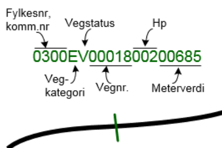
Figur 75: Vegreferansens oppbygning. Talleksemplet angir et punkt i Bispevika i Oslo.
