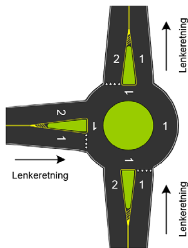
Figur 58: Rundkjøring med ett felt.
