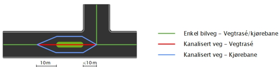
Figur 29: Avstanden fra hindringen til skillet mellom vegtrasé og kjørebane skal normalt sett være 10 meter.
