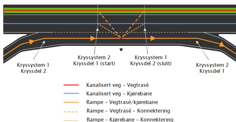
Figur 44: Metrering av vekslefelt
