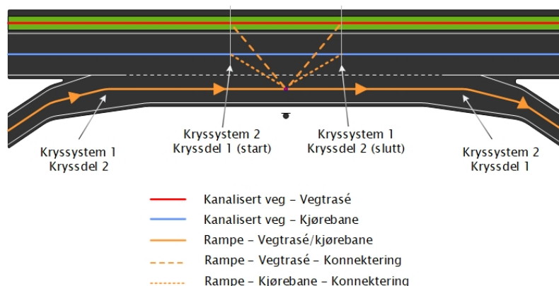
Figur 28: Geometri i vekslefelt
