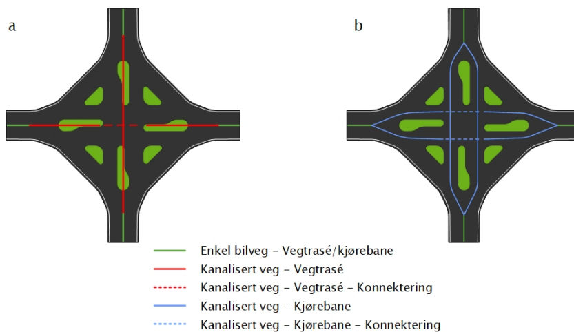
Figur 24: Geometri i kryss på vegtrasénivå (a) og geometri i kryss på kjørebanelnivå (b).
