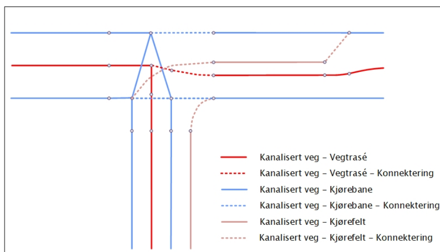
Figur 70: Vegtrasélenken skal normalt sett ligge midt mellom vegkantene, men i noen tilfeller må det gjøres lokale tilpasninger når lenken ellers vil komme i konflikt med lenker på detaljerte nivå.
