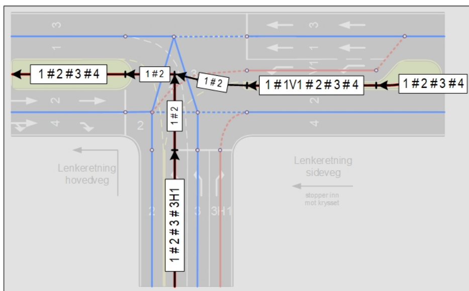
Figur 72: Oversikt over feltstrekningsojektets koding.
