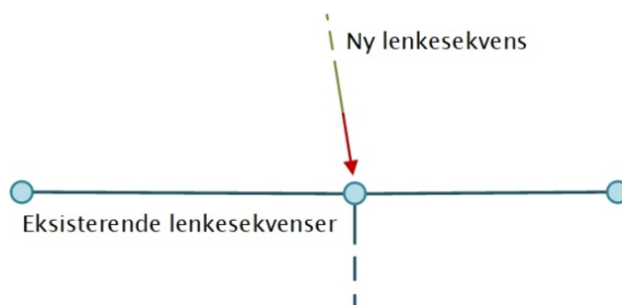
Figur 8: Tilkobling av ny veg til eksisterende T-kryss.
