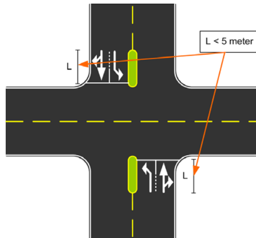
Figur 54: Oppmerkede felt kortere enn 5 meter registreres ikke, men inngår i hovedfeltet.
