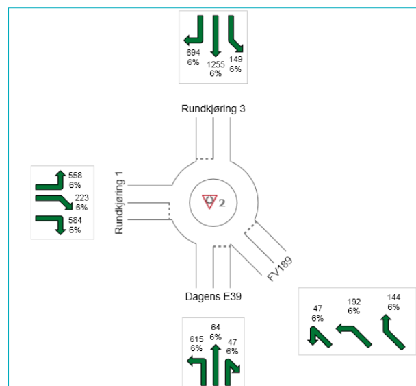
Figur 7: Trafikkttall for sørøstre rundkjøring i kryssprinsipp S1
