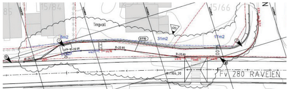
Opphøyd gangfelt ved Hotvedtveien
