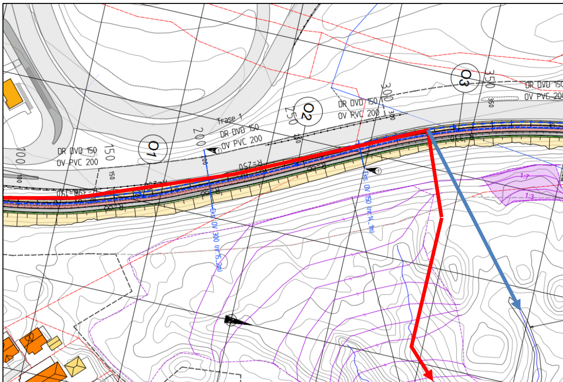
Figur 12. Flomvei (Rød pil = eksisterende flomvei, Blå pil = Ny flomvei ) Forslag til plassering av ny flomvei vist i figur 12 (Blå pil).
