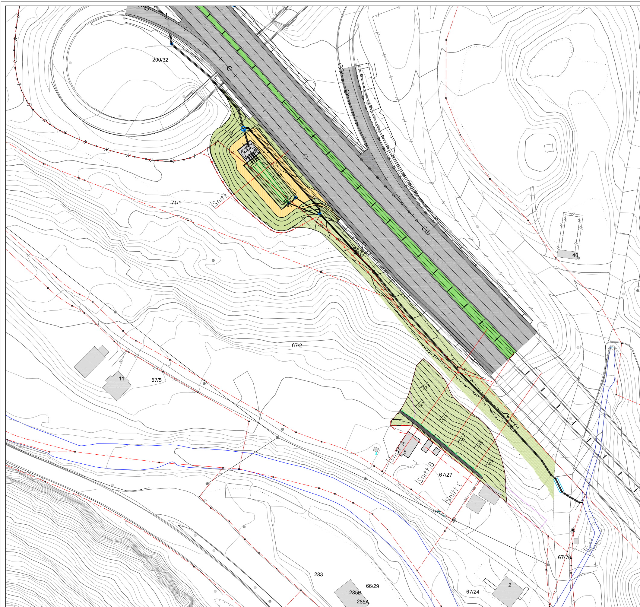
E16 Bjørum - Skaret Illustrasjonsplan rensedam og stabilitetstiltak
