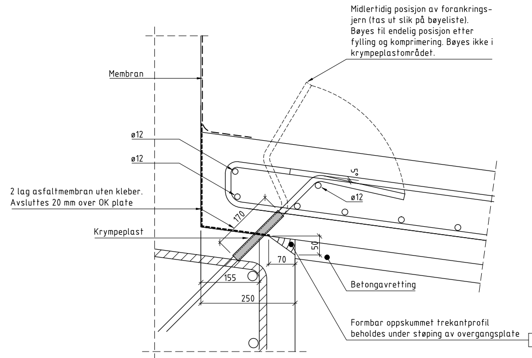
1 DETALJ 1:5
