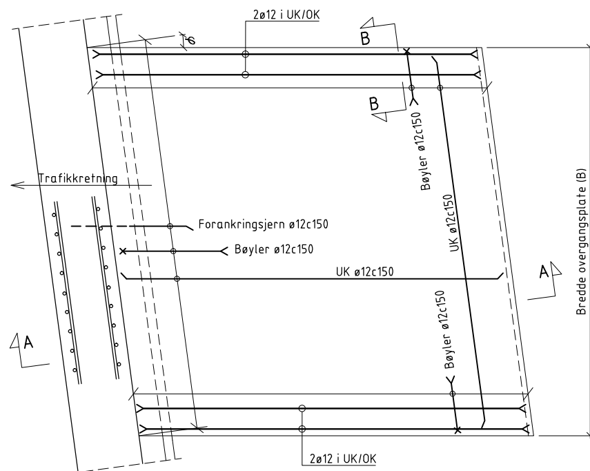
A PLAN: ARMERING VED SKJEVHET 0 < \tan \varphi \leq 0,25 1:20
