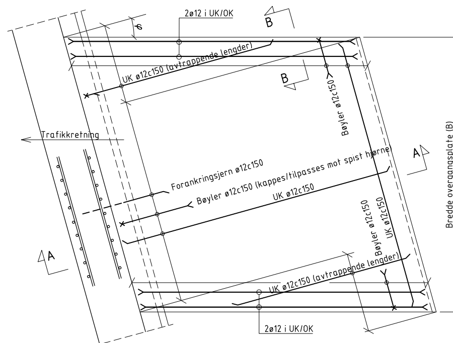
B PLAN: ARMERING VED SKJEVHET \tan \varphi > 0,25 1:20
