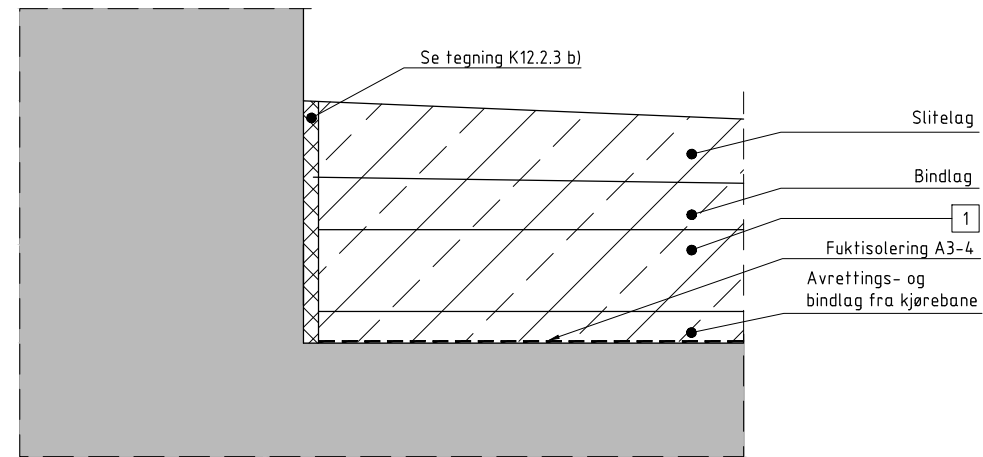
SNITT 1:5
