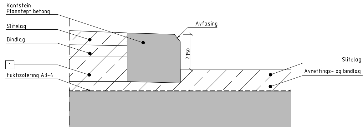
SNITT 1:5
