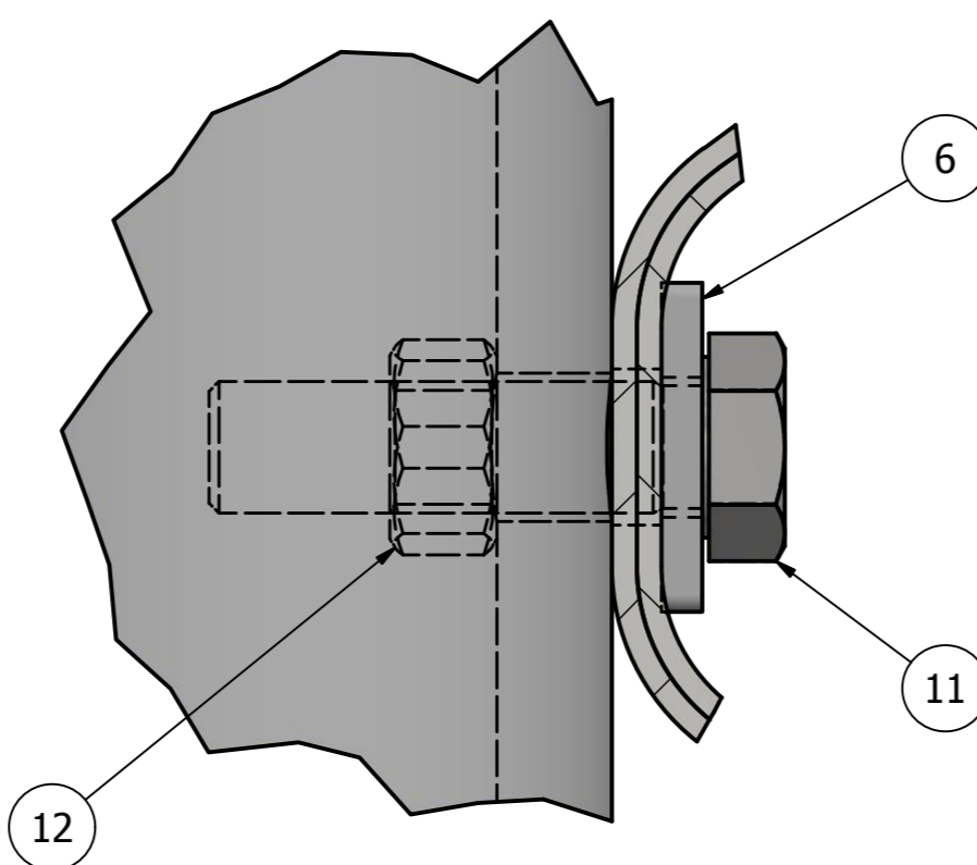
B (1 : 1)
