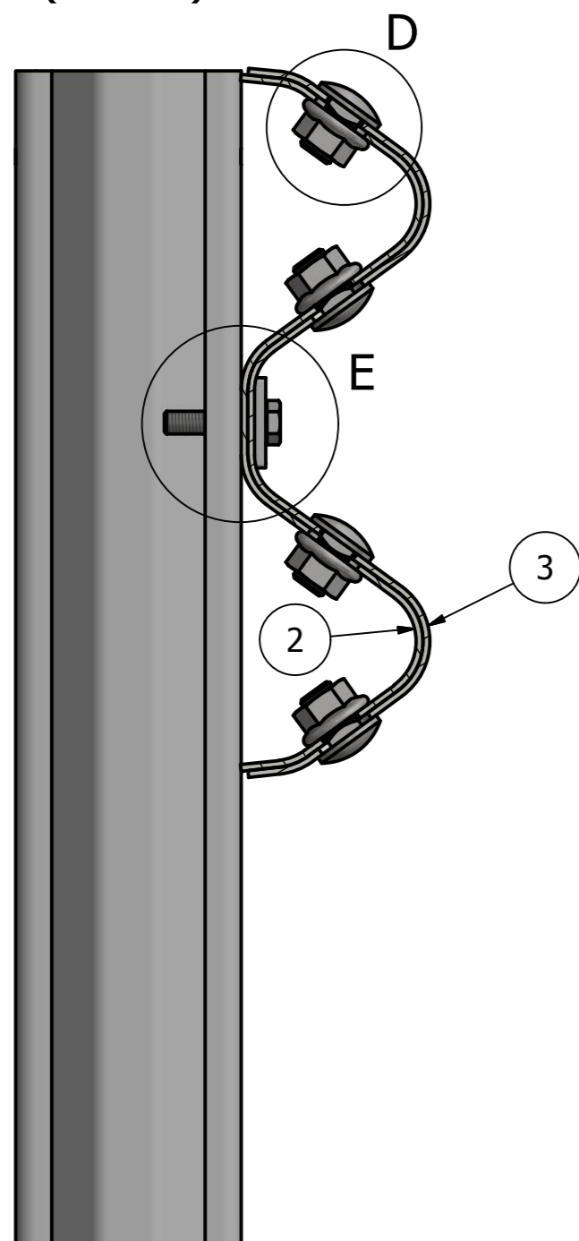
A-A (1:3)
