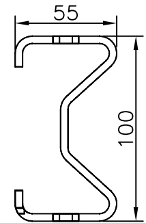
SNITT B:B
