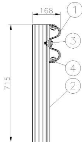
SNITT A:A
