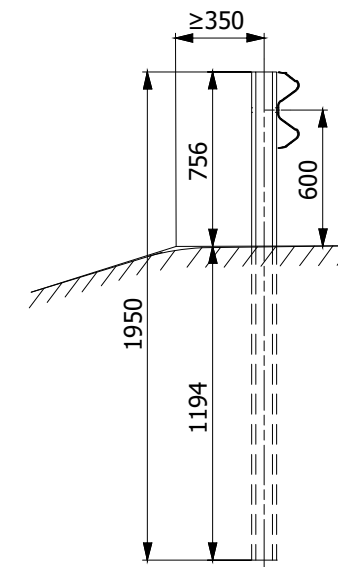
SEKTION A-A 1:20
