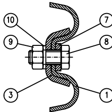
Snitt D
