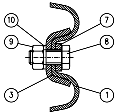
Snitt C
