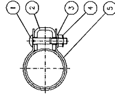
DETALJ 2 SKARV 1:2.5
