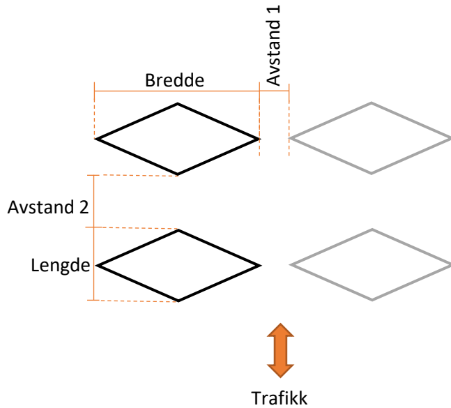
Figur 6. Skisse av S2-sensorer
