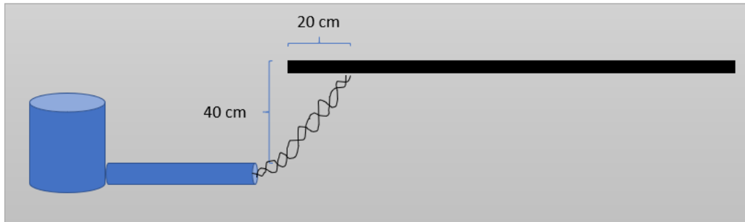
Figur 1. Nedføring av tilleder fra asfalt til trekkekum.
