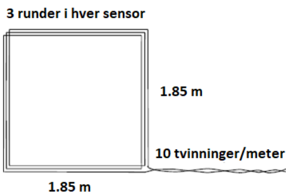
Figur 4. Riktig legging av leder for M1
