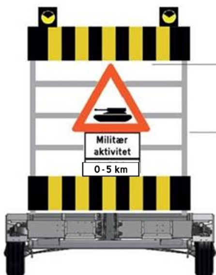
Figur 3 Varselpanel Militær aktivitet
