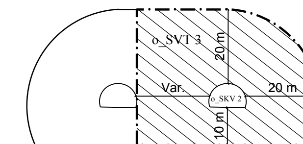
Tunnel med restriksjonssone. Snitt. o_SKV 2 - ny tunnel o_SVT 3 - restriksjonssone
