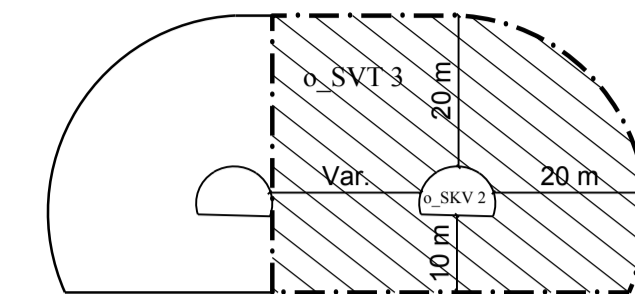
Tunnel med restriksjonszone. Snitt. o_SKV 2 - ny tunnel o_SVT 3 - restriksjonszone
