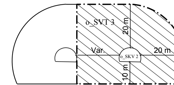
Tunnel med restriksjonssone. Snitt. o_SKV 2 - ny tunnel o_SVT 3 - restriksjonssone
