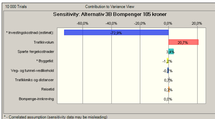
Figur 9 Usikkerhetsprofil for alternativ 3B
