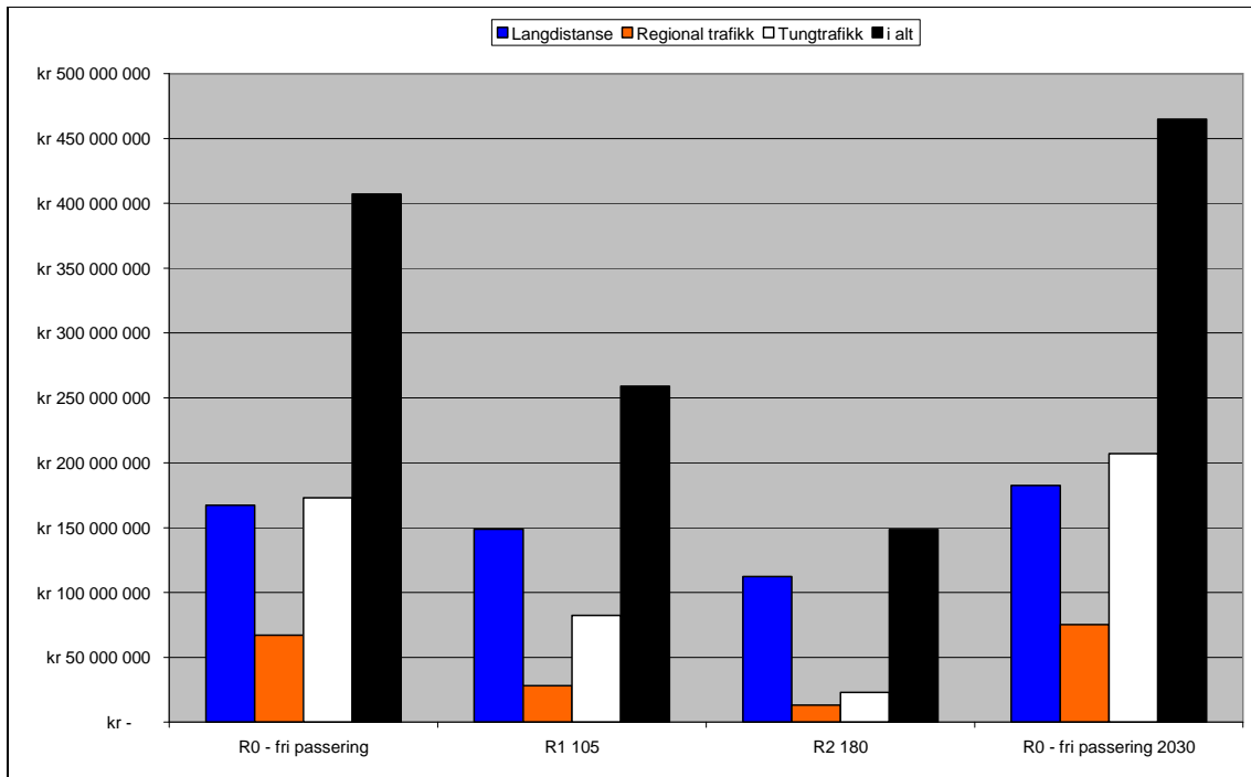
Figur 16 Årlig trafikantnytte og endringer i inntekter for bom- og fergeselskaper som følge av Rogfast etter alternativ
