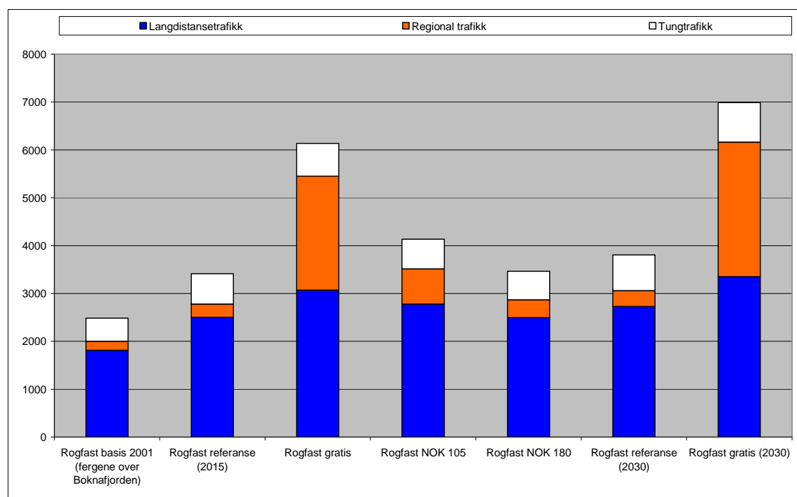
Figur 5 Trafikkvolumer (ÅDT) over Boknafjorden (Rogfast sør) etter trafikktype og alternativ
