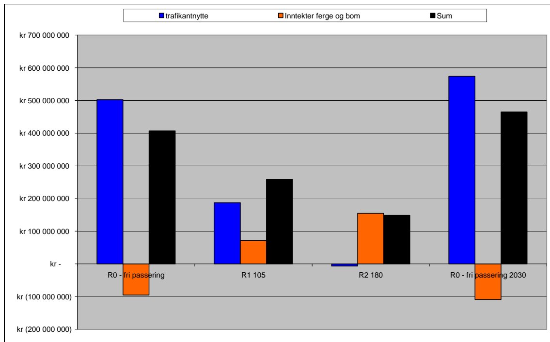
Figur 15 Årlig trafikantnytte og endringer i inntekter for bom- og fergeselskaper som følge av Rogfast etter trafikktype og alternativ
