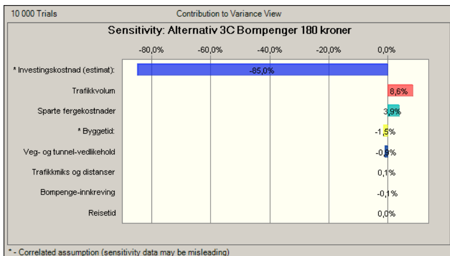
Figur 10 Usikkerhetsprofil for alternativ 3C
