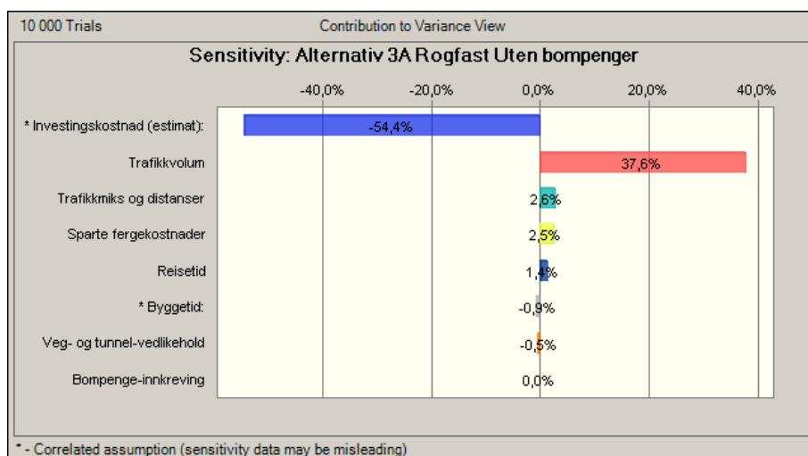
Figur 8 Usikkerhetsprofil for alternativ 3A
