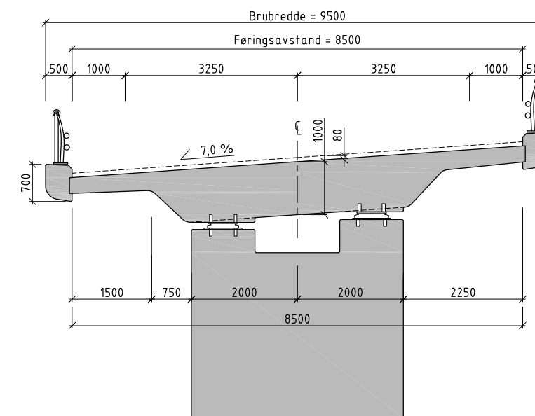
A SNITT 1:50
