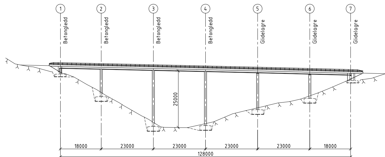
OPPRISS 1:500
