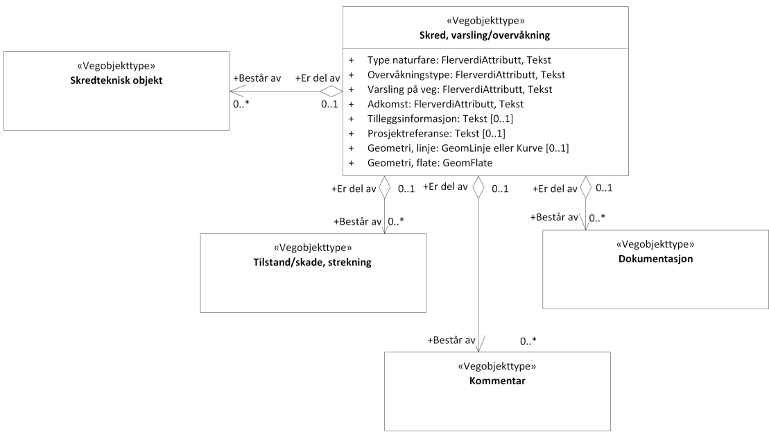
Figur 3: UML-skjema med assosiasjoner
