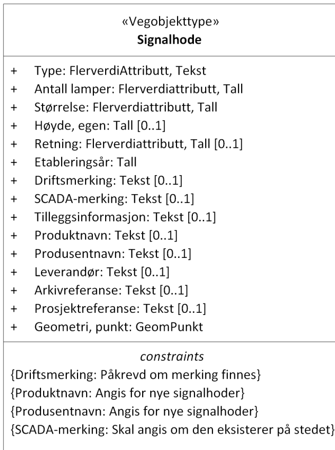
Figur 1: UML-skjema Signalhode
