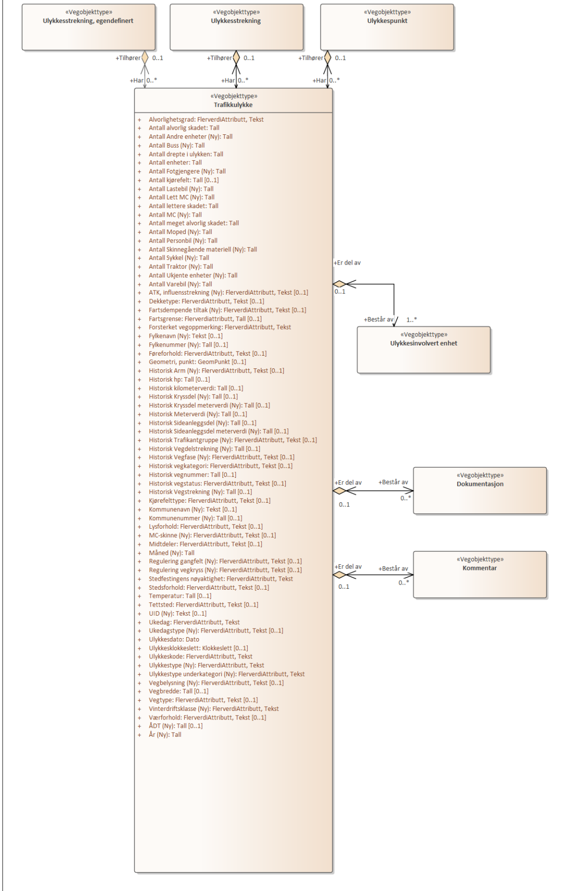
Figur 3: UML-skjema med assosiasjoner
